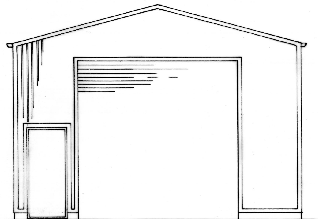
FRONTAGE 1:50
